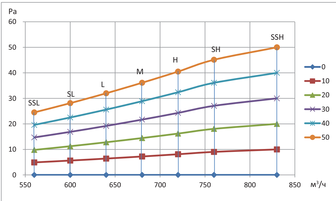
Рисунок 6.4: Производительность вентилятора блока MI2-56T2DN1
