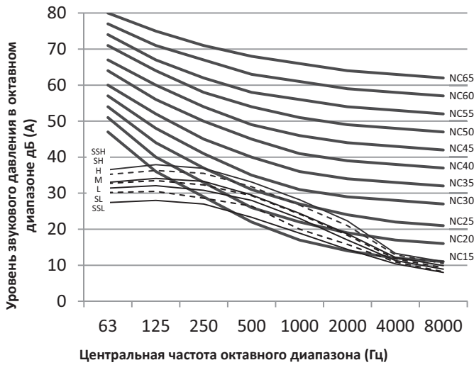
Рисунок 9.6: Уровни звукового давления в октавных полосах частот блока MI2-71T2DN1
