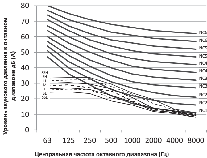
Рисунок 9.2: Уровни звукового давления в октавных полосах частот блока MI2-22(28)T2DN1
