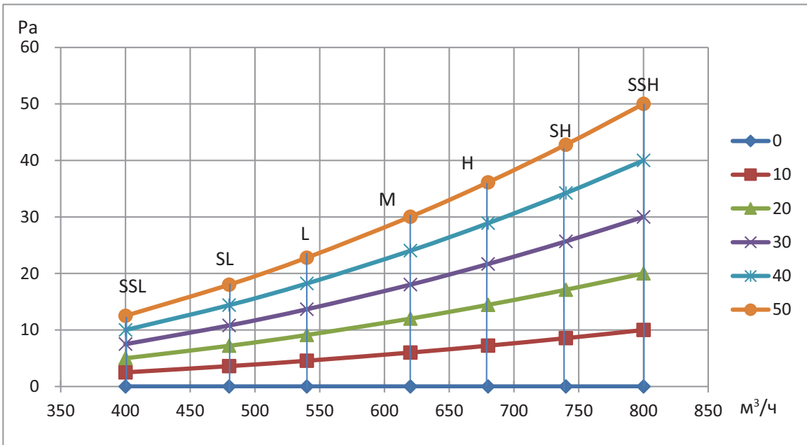
Рисунок 6.3: Производительность вентилятора блока MI2-45T2DN1
