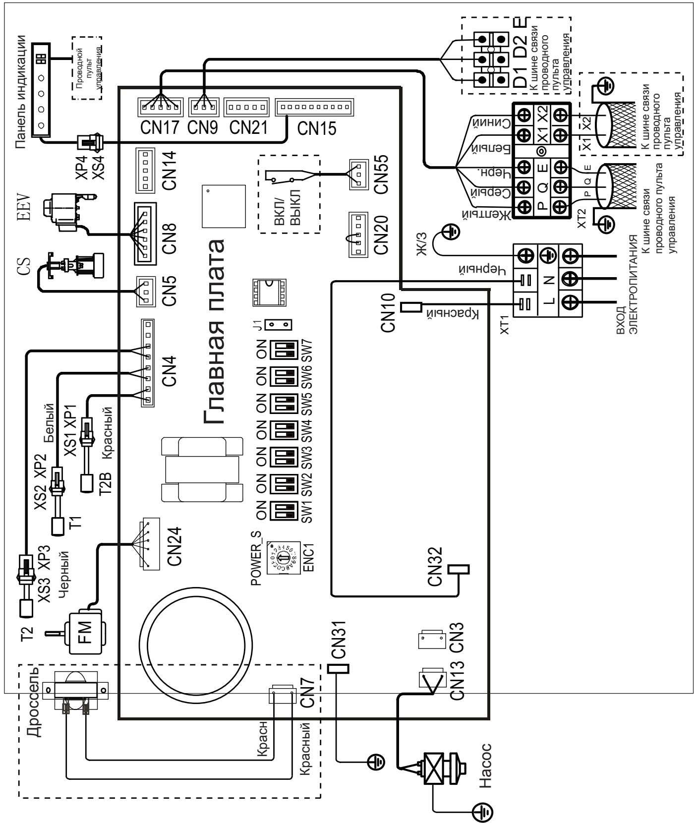
Рисунок 5.1: Электрическая схема средненапорного канального блока
