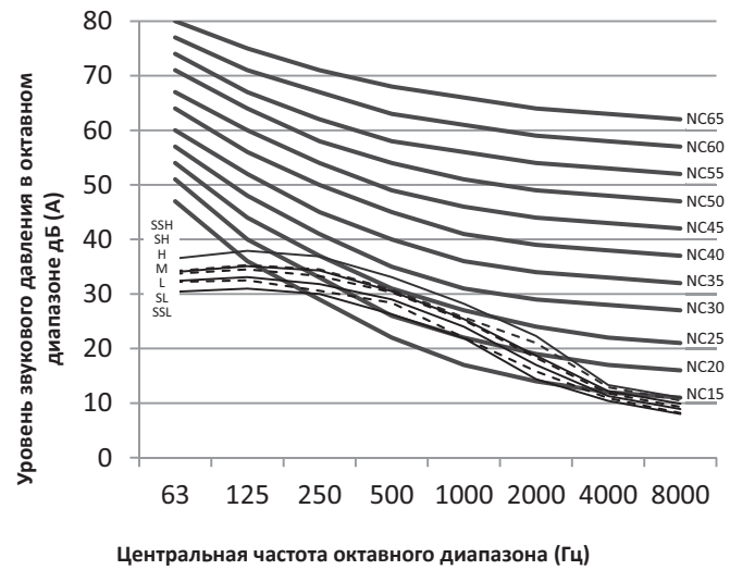
Рисунок 9.5: Уровни звукового давления в октавных полосах частот блока MI2-56T2DN1
