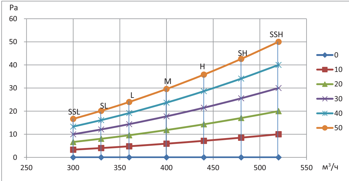
Рисунок 6.1: Производительность вентилятора блока MI2-22(28)T2DN1
