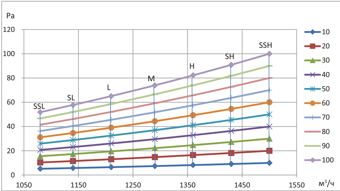
Рисунок 6.7: Производительность вентилятора блока MI2-112T2DN1
