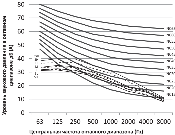
Рисунок 9.8: Уровни звукового давления в октавных полосах частот блока MI2-112T2DN1
