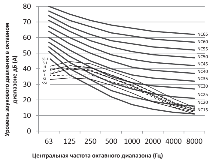
Рисунок 9.9: Уровни звукового давления в октавных полосах частот блока MI2-140T2DN1
