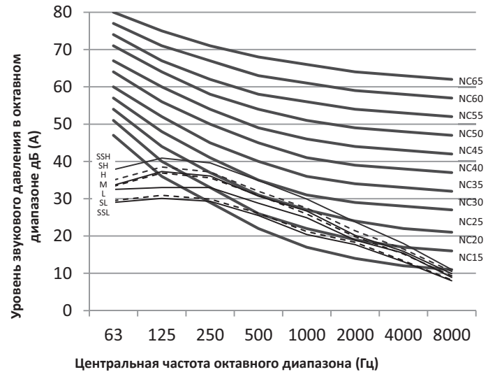
Рисунок 9.7: Уровни звукового давления в октавных полосах частот блока MI2-80(90)T2DN1
