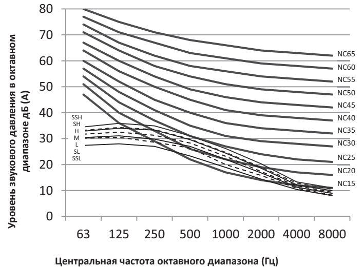
Рисунок 9.3: Уровни звукового давления в октавных полосах частот блока MI2-36T2DN1
