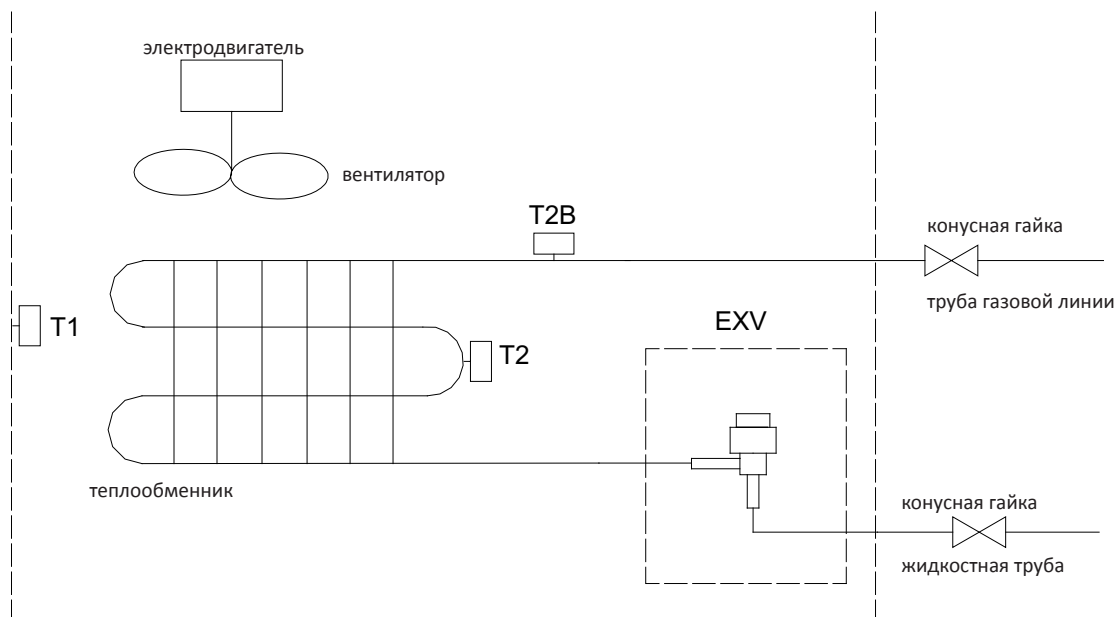
Рисунок 4.1: Схема трубопроводов средненапорного канального блока
