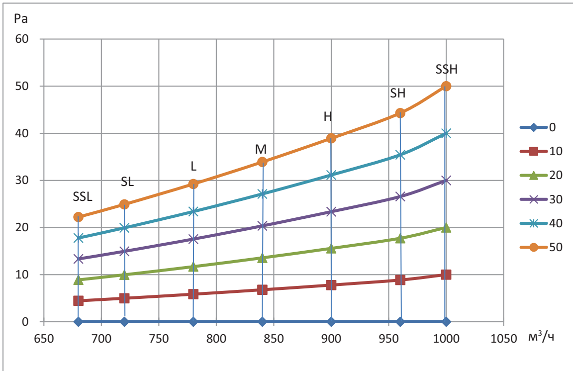
Рисунок 6.5: Производительность вентилятора блока MI2-71T2DN1
