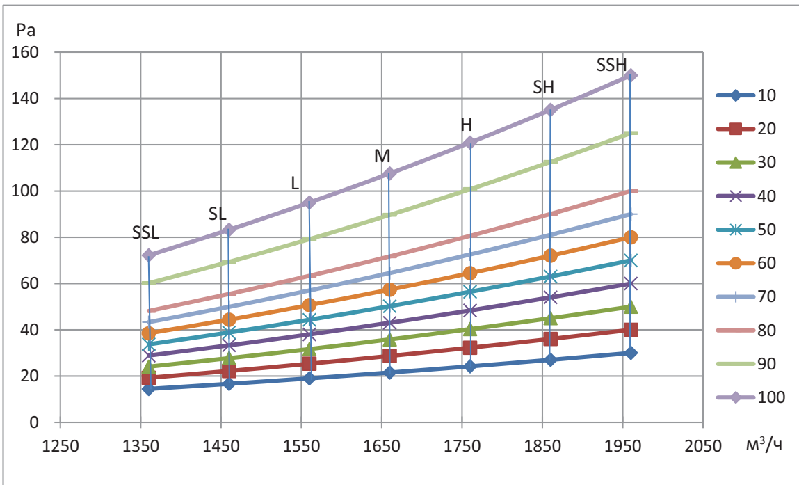
Рисунок 6.8: Производительность вентилятора блока MI2-140T2DN1
