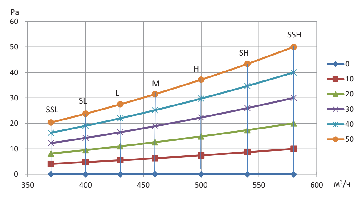
Рисунок 6.2: Производительность вентилятора блока MI2-36T2DN1
