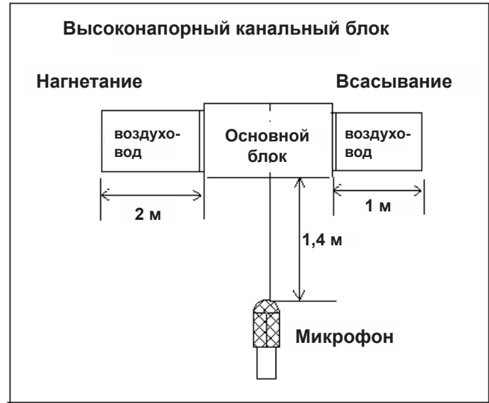
Рисунок 9.1: Измерение уровня звукового давления средненапорного канального блока
