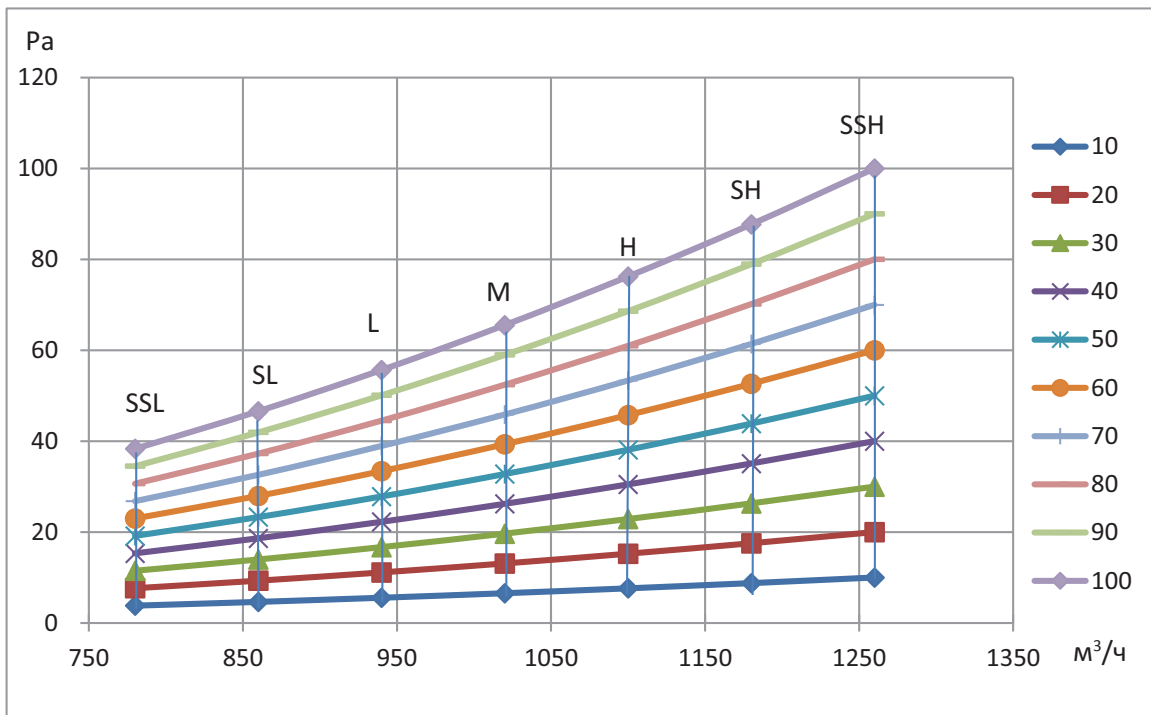
Рисунок 6.6: Производительность вентилятора блока MI2-80(90)T2DN1
